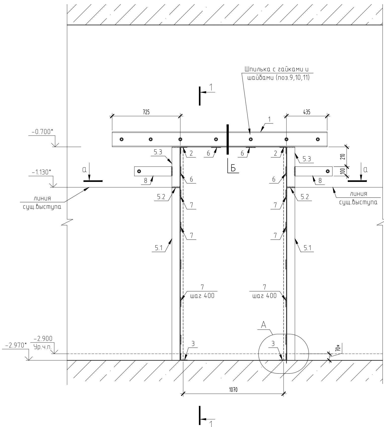
Обетонировать по се Ø5 Вр-1, яч.50х50
